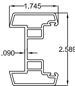
40 ASTRAGAL
