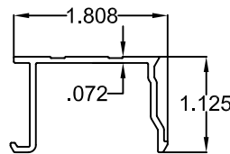
4 FRAME CAP
